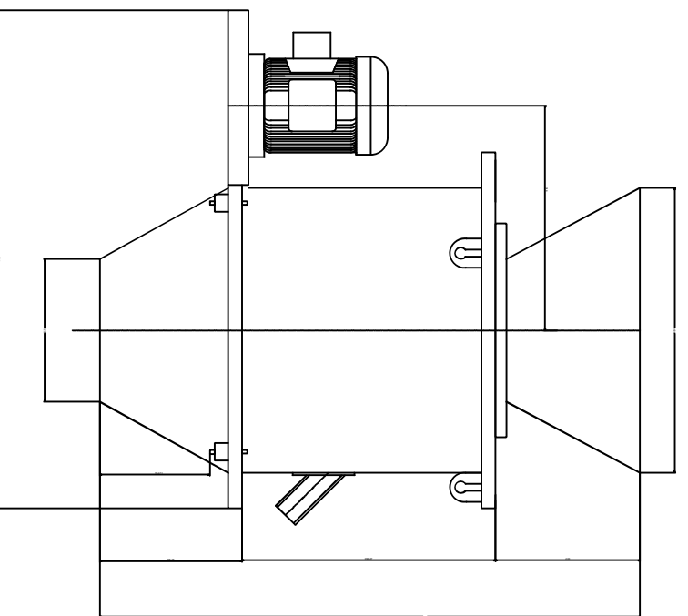
MODEL:AL-150
